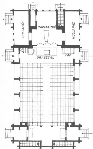
FÖLDSZINTI ALAPRAJZ
