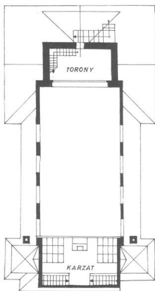
KARZAT ALAPRAJZ
