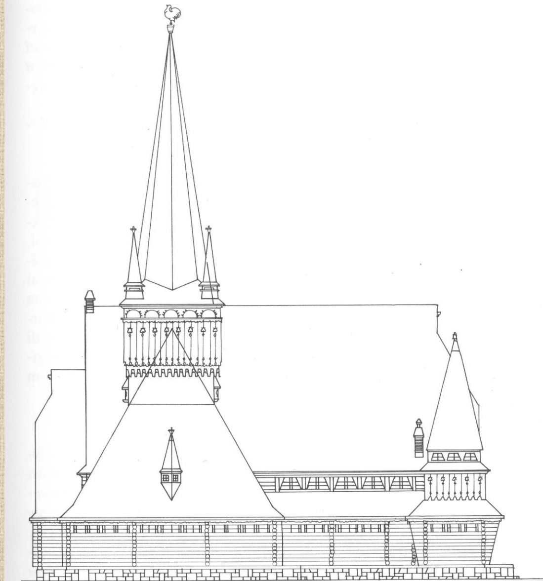
DÉLI HOMLOKZAT
