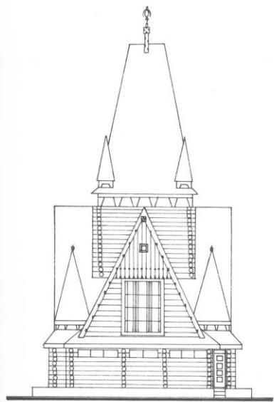
FŐHOMLOKZAT
